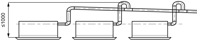
T-eklemlili birleşen tahliye boruları
